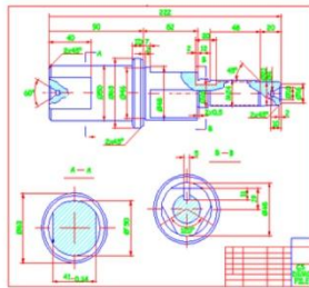
Vektorisierungsergebnis
